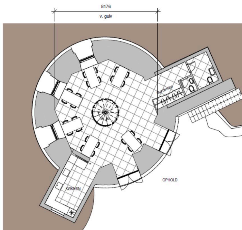
Plan af møllebase
